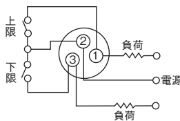
結線図
