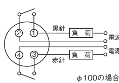
結線図
