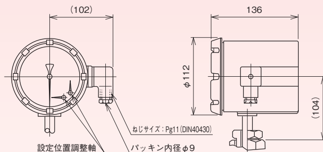
外形寸法
