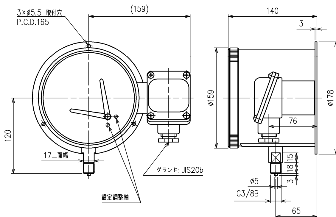
JM22 (丸縁形 接点付圧力スイッチ)
