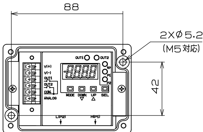
<図 7-1 取付方法>
